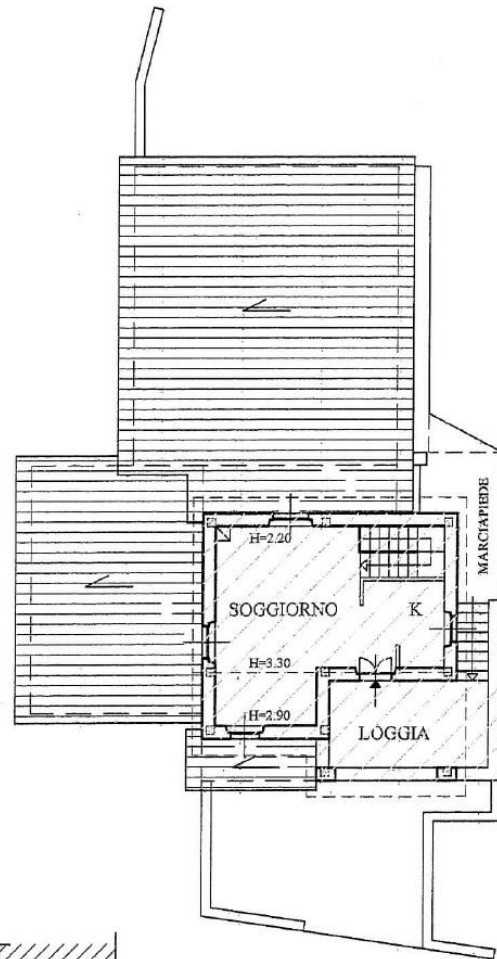
PIANO PRIMO
