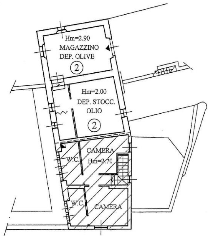
PIANO PRIMO
