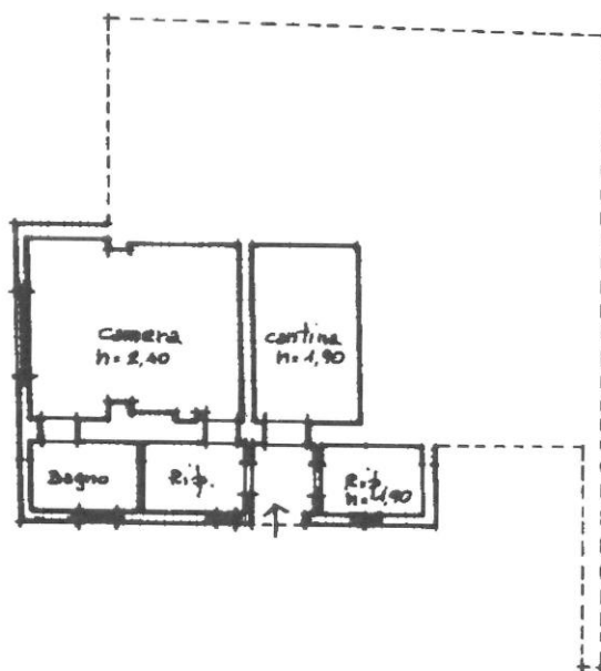
PIANO 1° SEMINTERRATO
