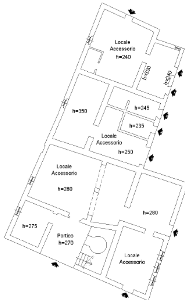
PIANTA PIANO TERRENO
