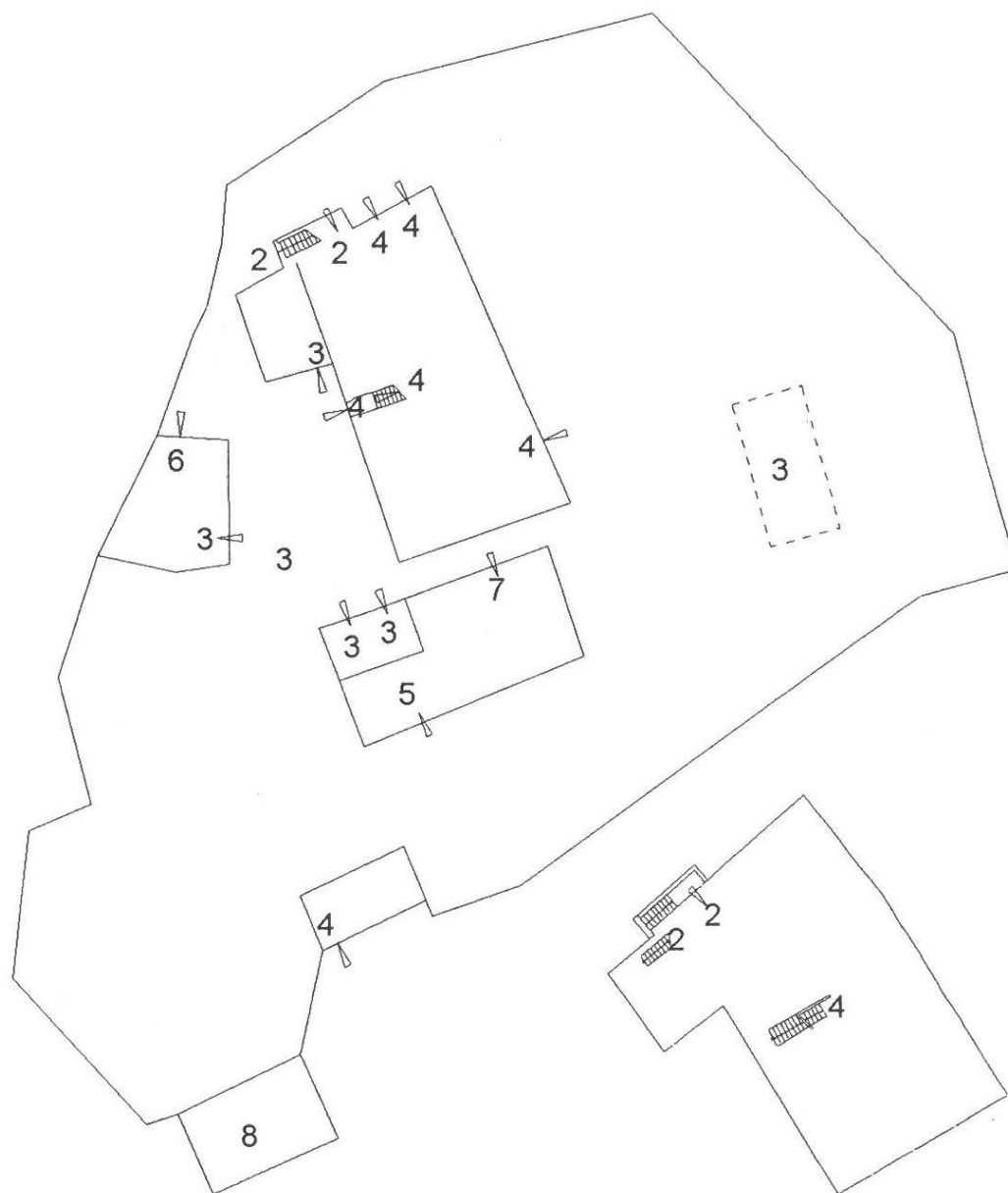
PIANO PRIMO
